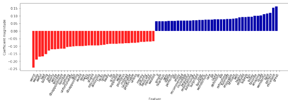
Figure: 係数が最大/最小である特徴量
